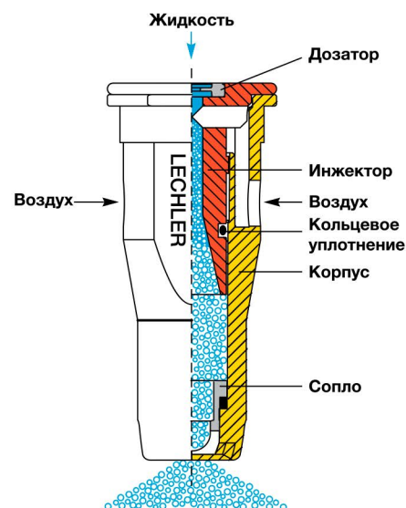
Съемный инжектор
